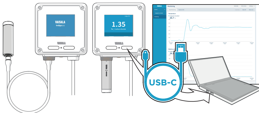
图 22 探头连接选项
