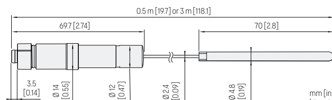
TMP115 dimensions
