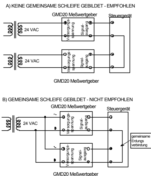
Abbildung 5 AC Anschluß an eine AC-Versorgung
