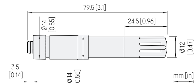
HMP115 dimensions
