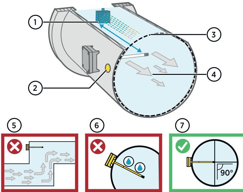
Figure 23 Présentation de l'installation sur conduite
