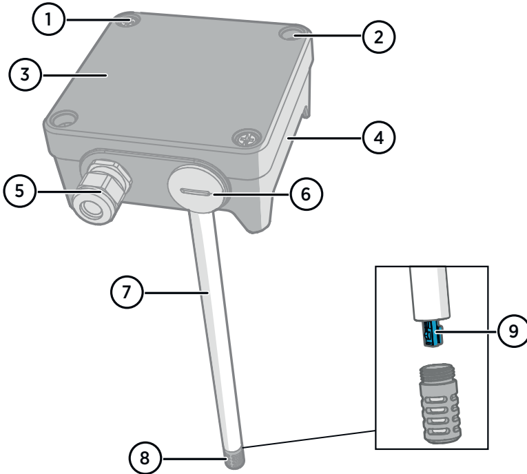
图 71 HMD62 和 TMD62 变送器部件概览
