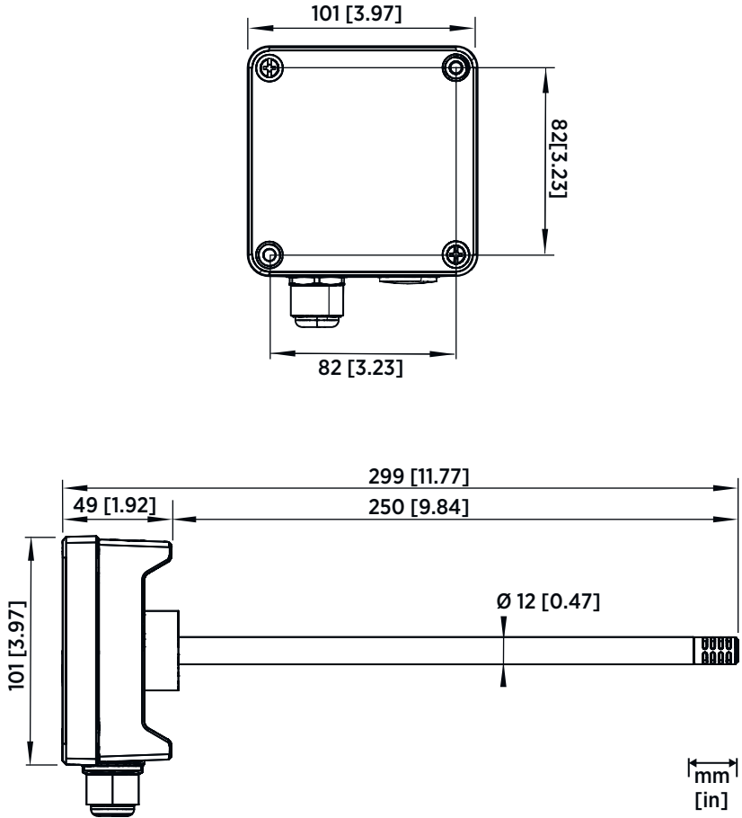
Figura 32 Dimensiones de HMD60
