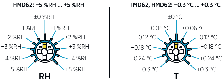
Figure 29 Plages de réglage des condensateurs HR et T (indicatives)
