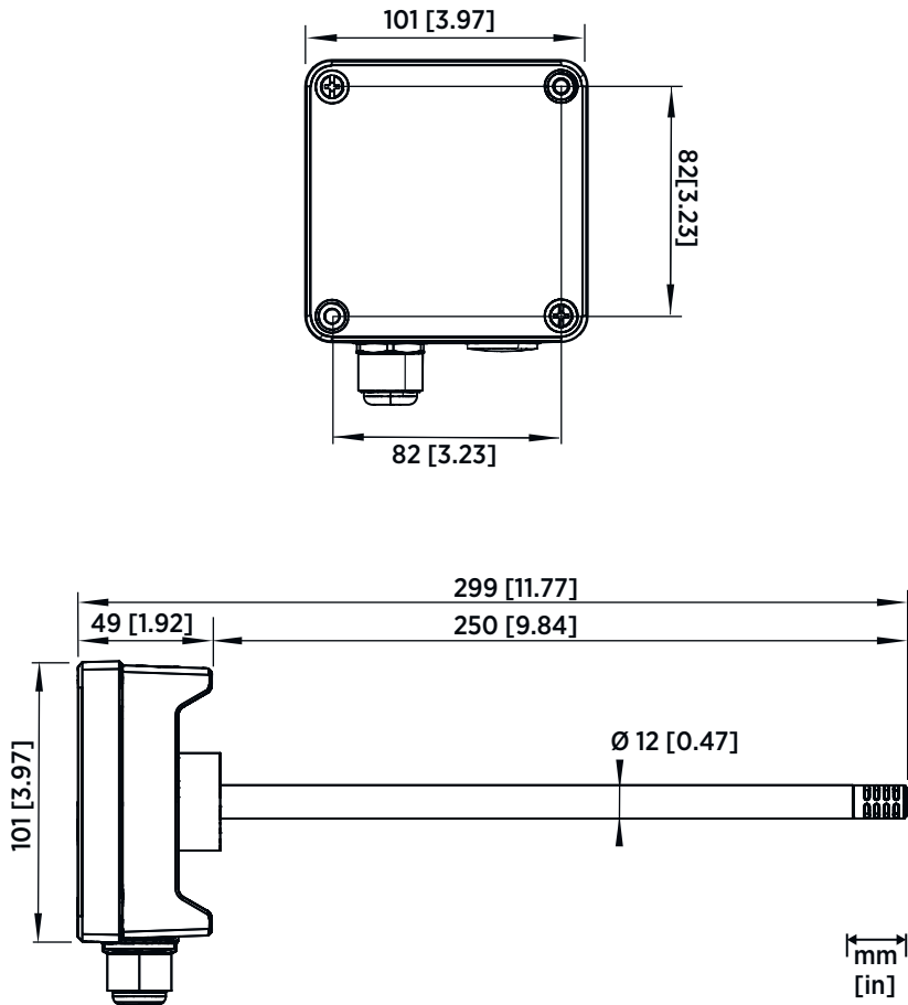
Figura 42 Dimensões do HMD60
