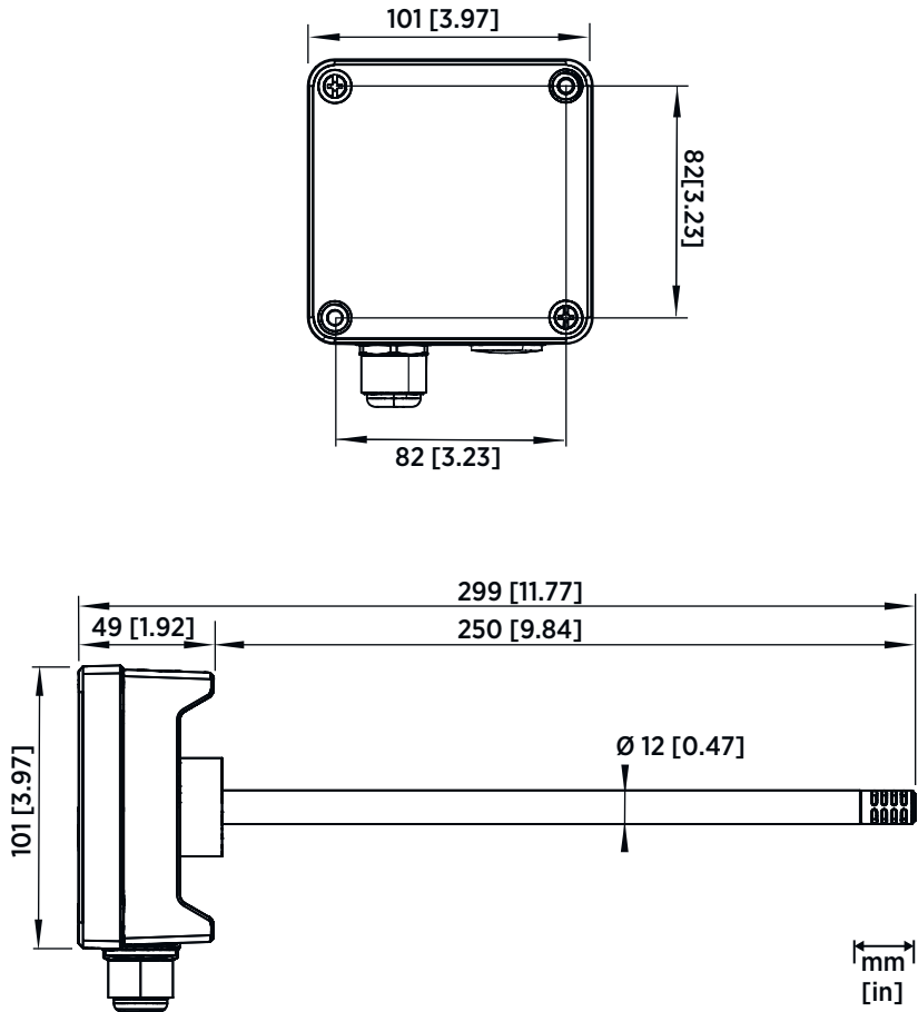
Abbildung 12 Abmessungen HMD60
