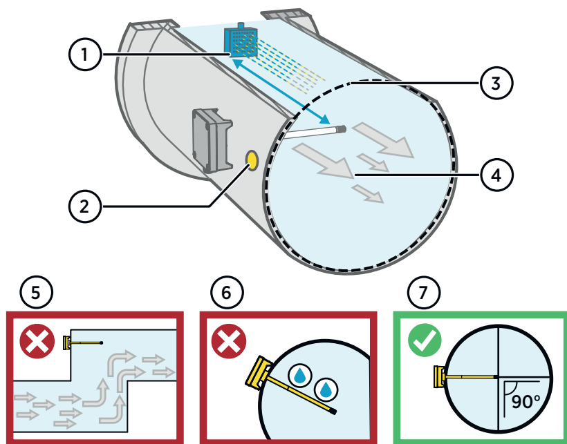
Рис. 53 Общие сведения об установке в воздуховод
