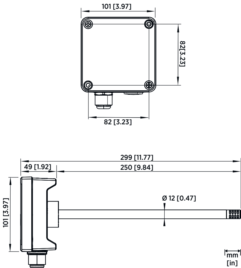
Рис. 52 Размеры HMD60
