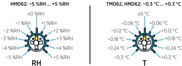
Abbildung 19 rF- und T-Trimmereinstellungsbereiche (Anhaltswert)
