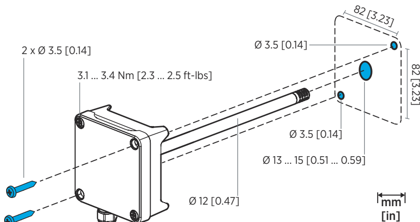
Figura 44 Inserir e montar parafusos
