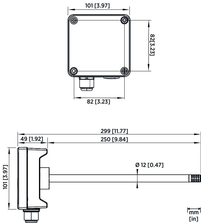
図 62 HMD60 の寸法
