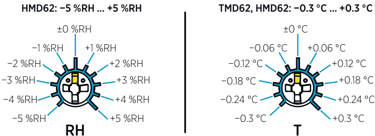
Figura 39 Rangos de ajuste de la cortadora de HR y T (indicativo)
