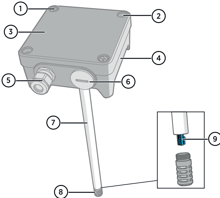
Figure 21 Présentation des pièces des transmetteurs HMD62 et TMD62
