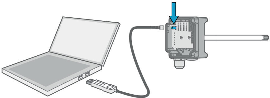
Abbildung 17 Verbindung des Messwertgebers mit Insight
